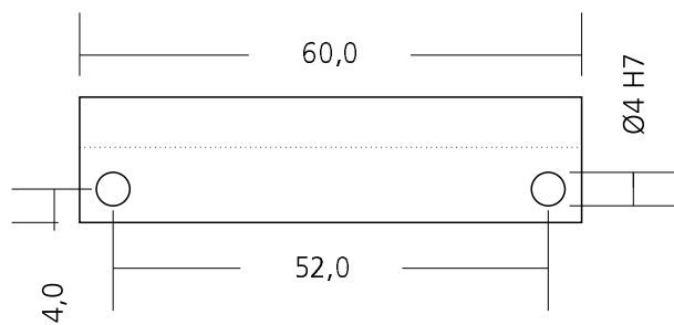
Aufspannblock (Aluminium)
